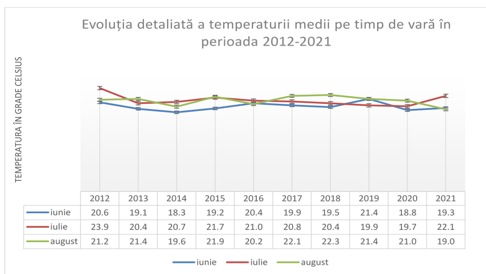
Figura 2.5 Evoluția detaliată a temperaturii medii pe timp de vară în perioada 2012-2021 (ANM, 2022)
