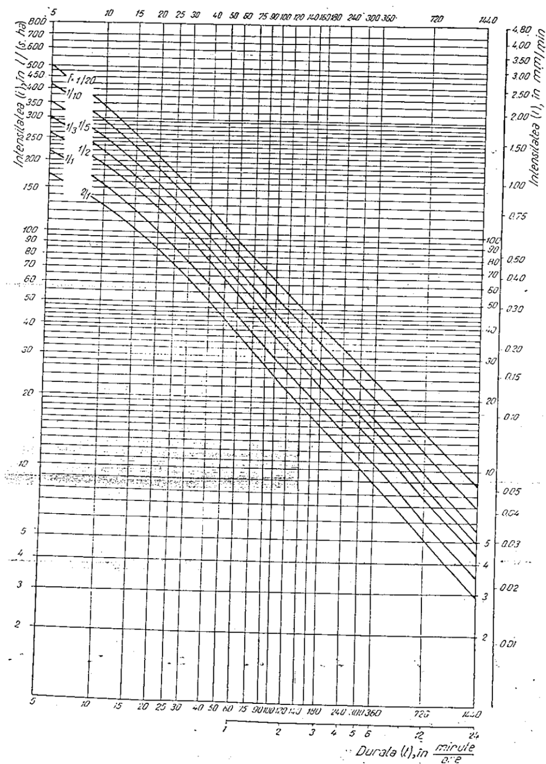
Imagine 5.2 Diagramme ploi maxime zona 16
