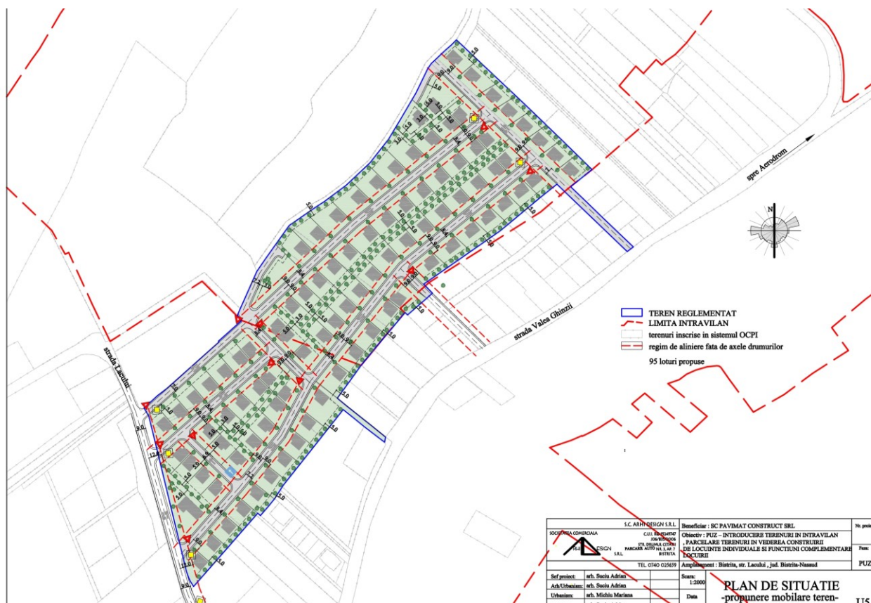
FIGURA 23. PUZ STR. LACULUI - PLAN DE MOBILARE
