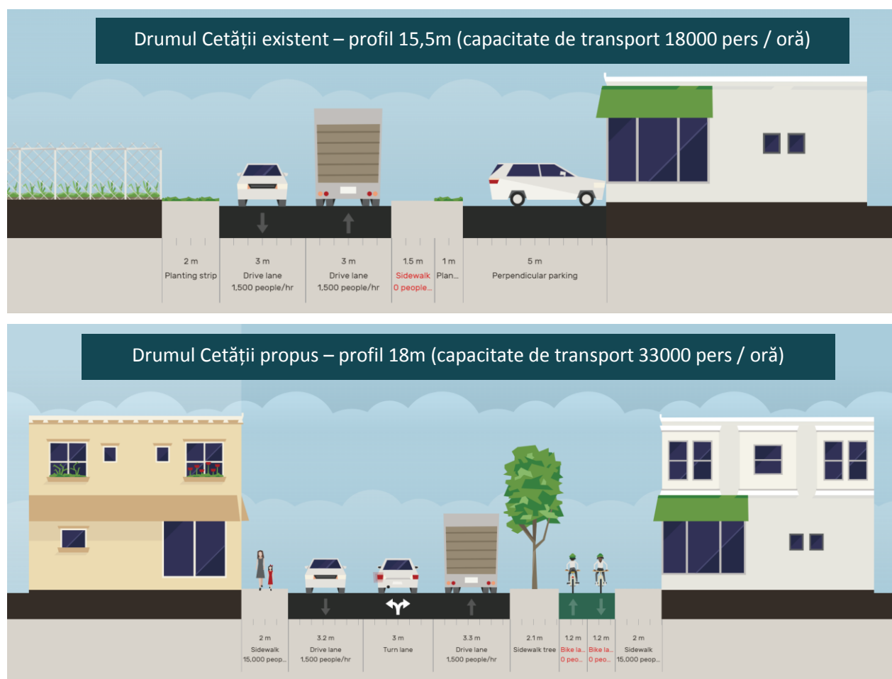
FIGURA 148 ILUSTRARE SECȚIUNE CARACTERISTICĂ DRUMUL CETĂȚII (EXISTENT-PROPOS)
