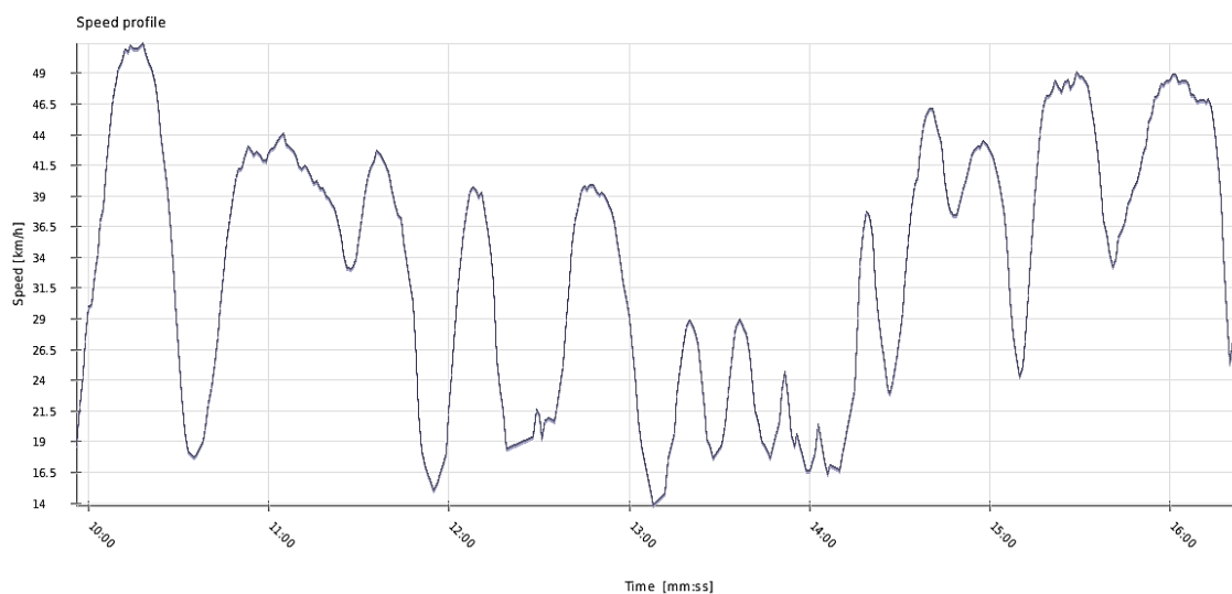
FIGURA 88. VARIAȚIA VITEZEI DE-A LUNGUL TRASEULUI 3 (VERDE) SENS SUBCETATE – VALEA JELNEI
