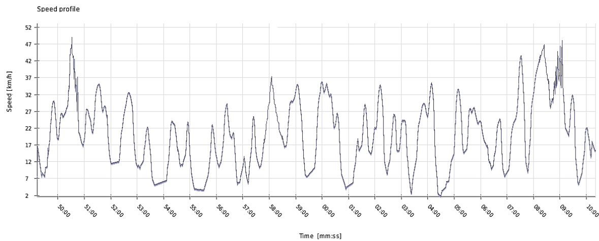
FIGURA 93. VARIAȚIA VITEZEI DE-A LUNGUL LINIEI 3 SENS CR VIVU – DRUMUL CETĂȚII
