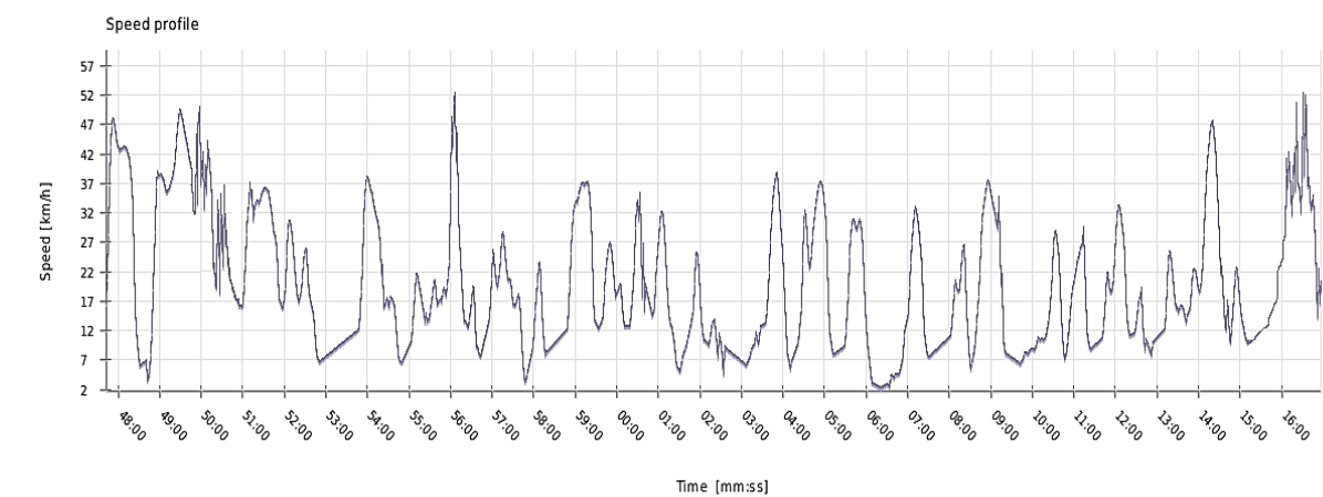
FIGURA 90. VARIAȚIA VITEZEI DE-A LUNGUL LINIEI 2 SENS VIIȘOARA - UNIREA
