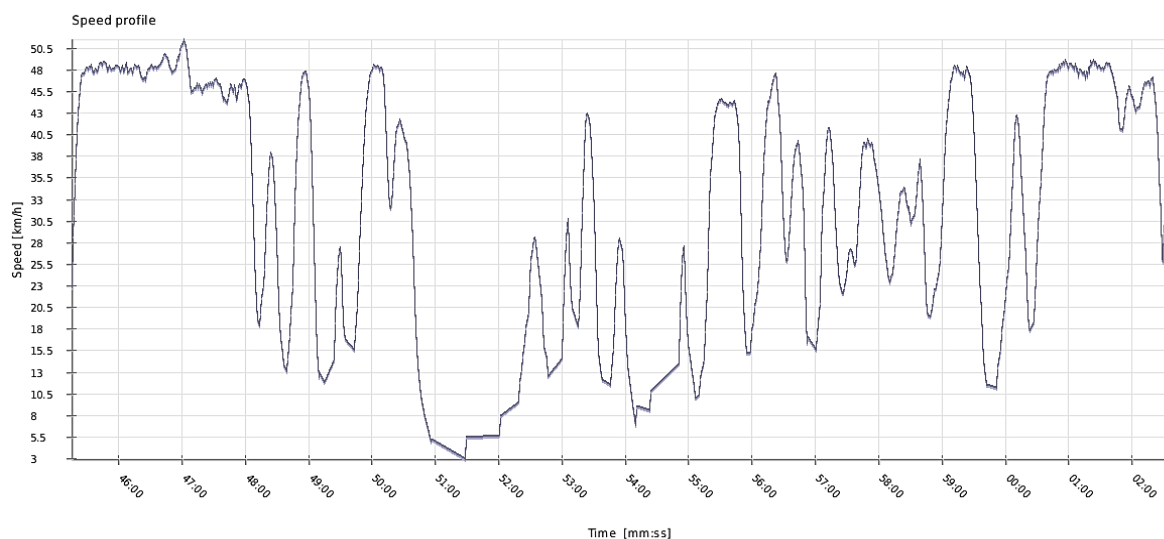
FIGURA 85. VARIAȚIA VITEZEI DE-A LUNGUL TRASEULUI 2 (ROȘU) SENS VIȘOARA – UNIREA
