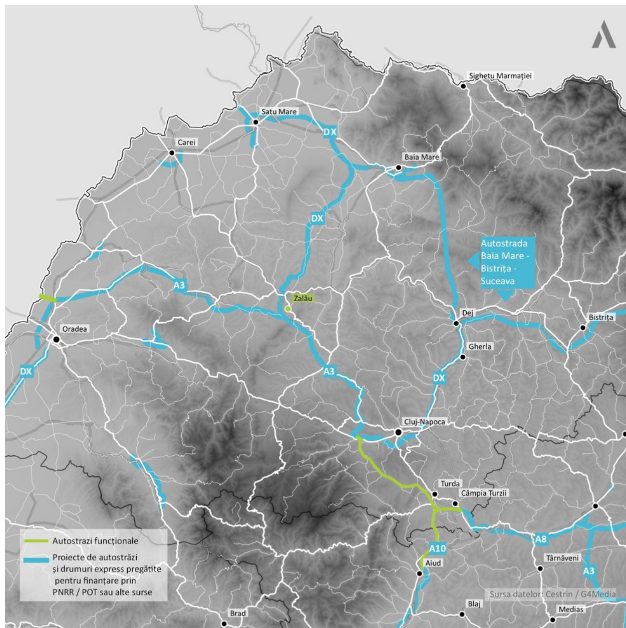
FIGURA 30. PROIECTELE DE INFRASTRUCTURĂ RUTIERĂ MAJORĂ PLANIFICATE ÎN REGIUNEA NORD-VEST
