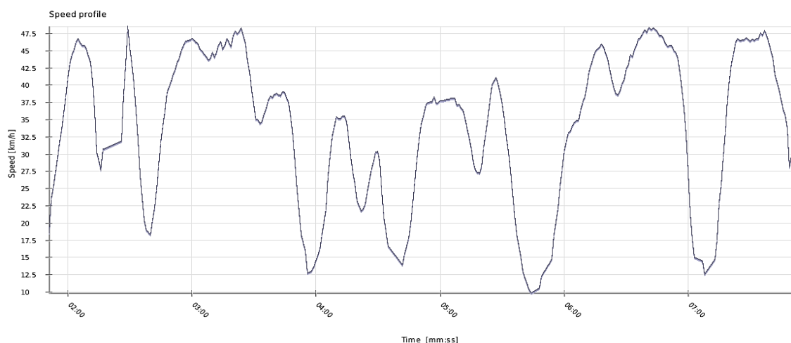
FIGURA 87. VARIAȚIA VITEZEI DE-A LUNGUL TRASEULUI 3 (VERDE) SENS VALEA JELNEI - SUBCETATE
