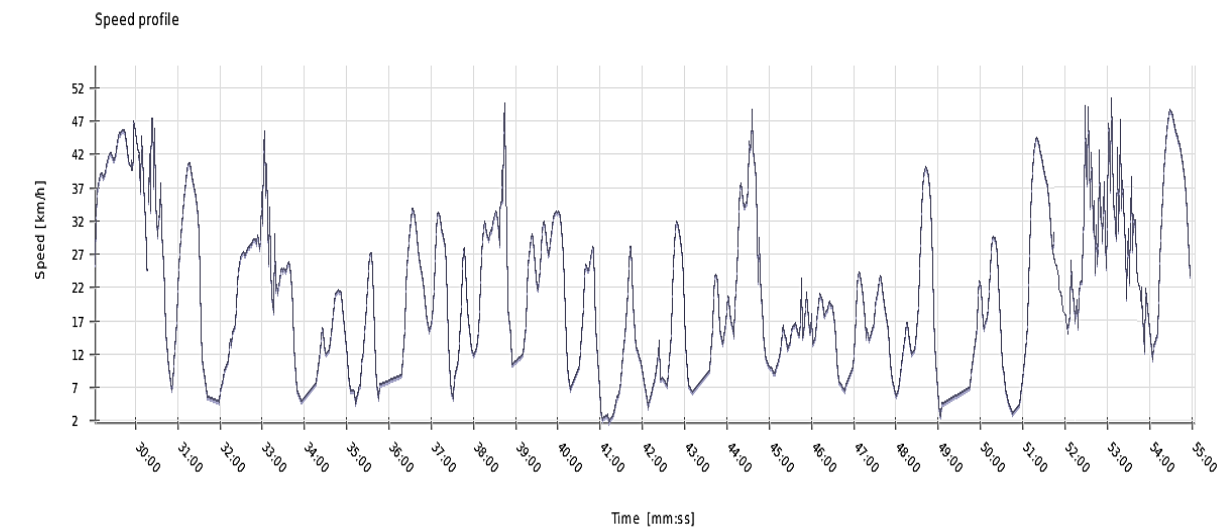
FIGURA 91. VARIAȚIA VITEZEI DE-A LUNGUL LINIEI 2 SENS UNIREA – VIIȘOARA
