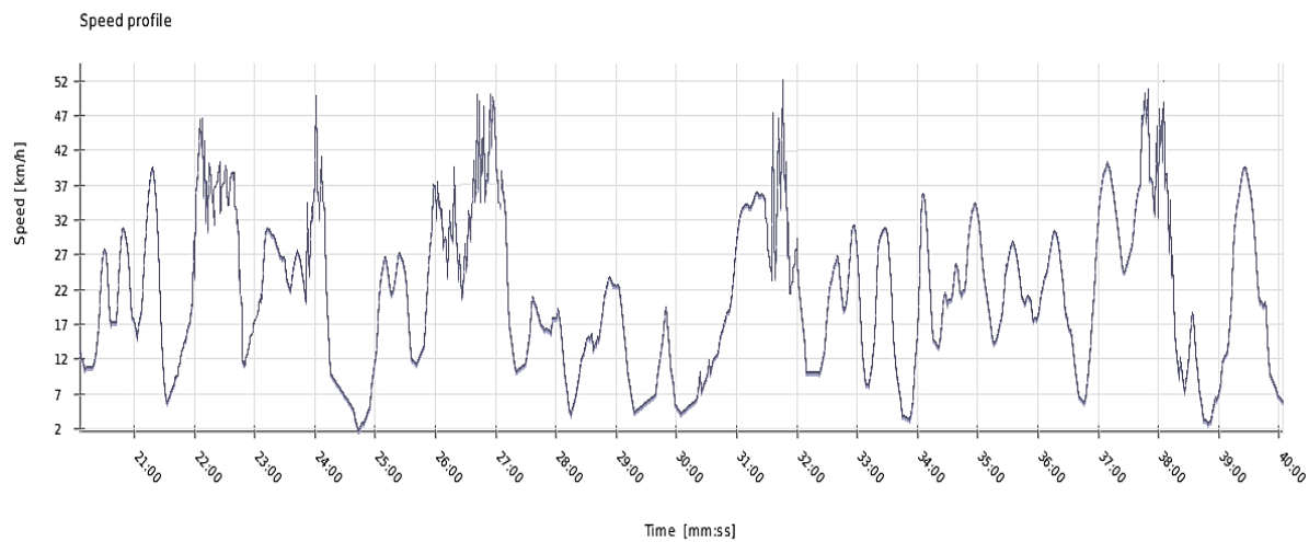
FIGURA 92. VARIAȚIA VITEZEI DE-A LUNGUL LINIEI 3 SENS DRUMUL CETĂȚII – CR VIVU
