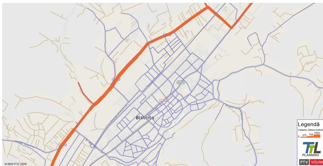
FIGURA 108. MĂRIMEA FLUXURILOR DE TRAFIC – VEHICULE GRELE DE MARFĂ – AN DE BAZĂ 2021
