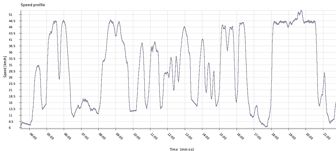
FIGURA 86. VARIAȚIA VITEZEI DE-A LUNGUL TRASEULUI 2 (ROȘU) SENS UNIREA – VIȘOARA
