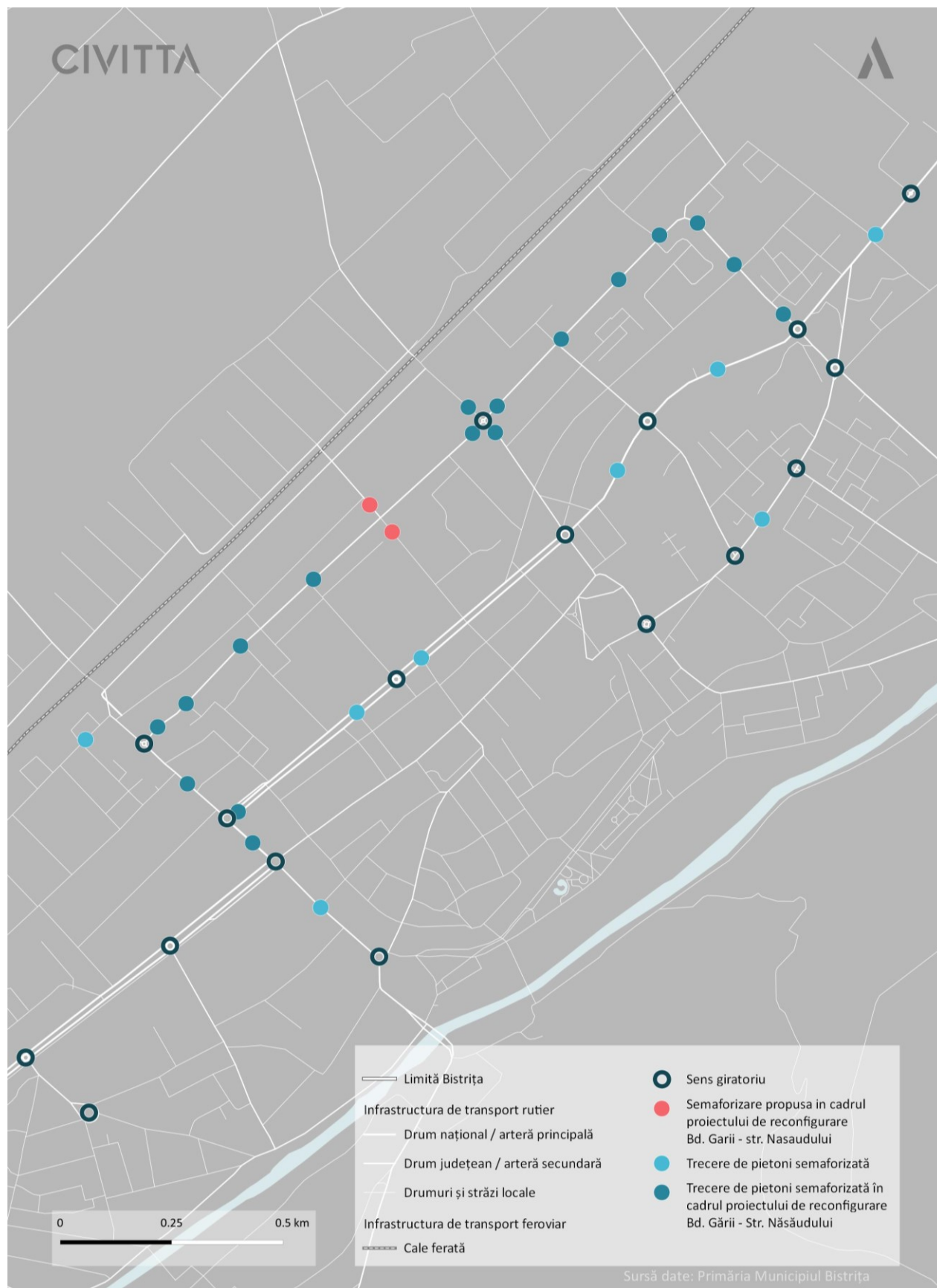
FIGURA 49 SISTEMUL DE MANAGEMENT AL TRAFICULUI LA NIVELUL ZONEI CENTRALE
