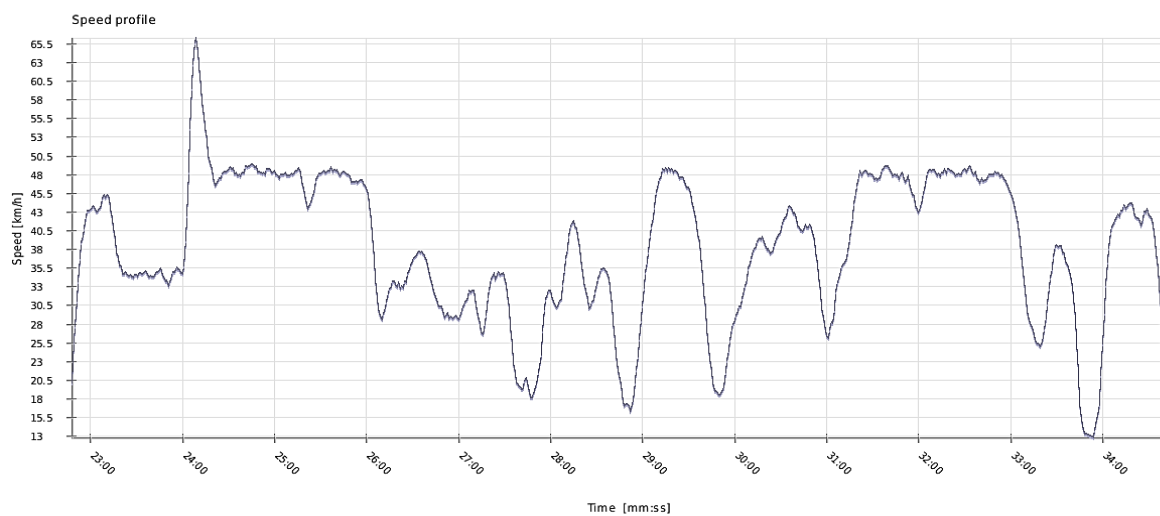
FIGURA 83. VARIAȚIA VITEZEI DE-A LUNGUL TRASEULUI 1 (ALBASTRU) SENS VIȘOARA – CALEA MOLDOVEI
