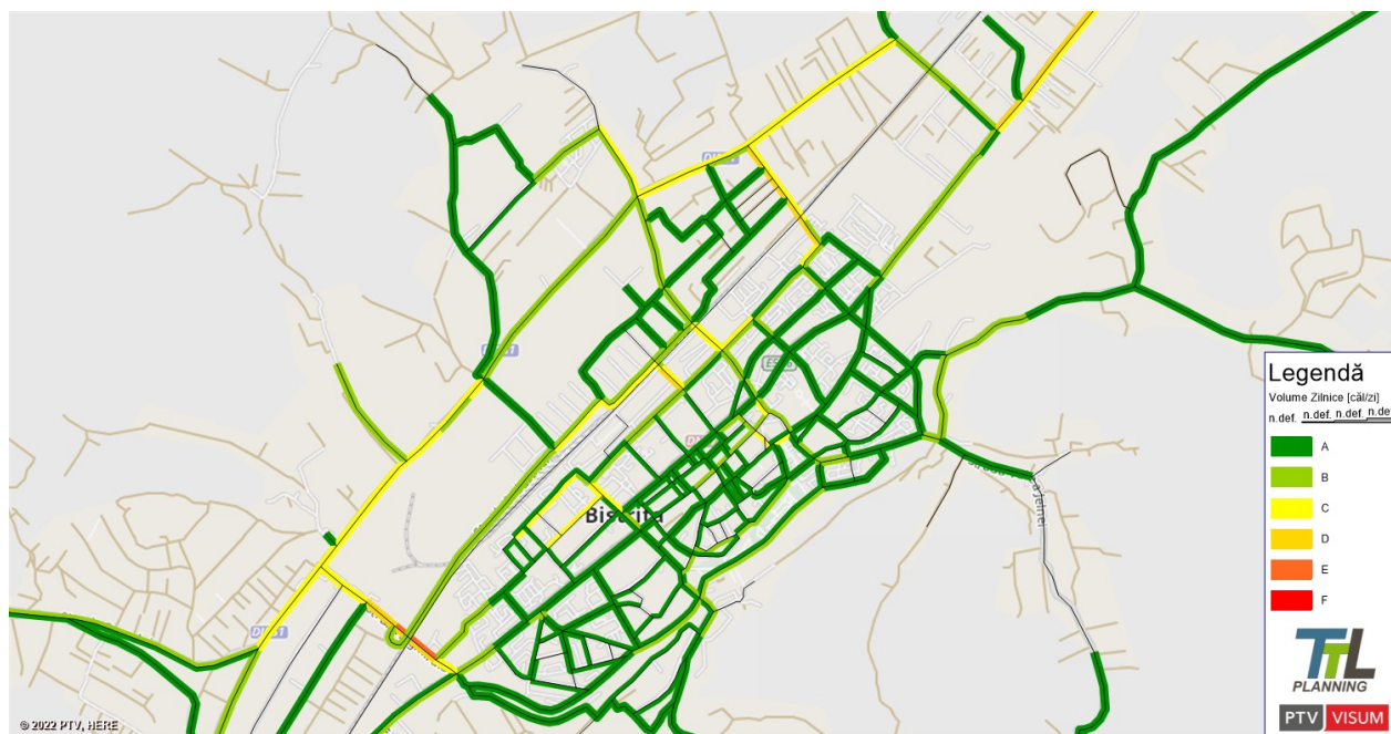
FIGURA 135. NIVELUL DE SERVICIU AL REȚELEI RUTIERE – AN DE PROGNOZĂ 2035
