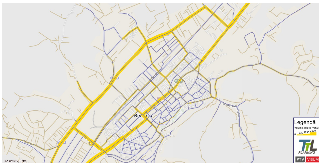
FIGURA 106. MĂRIMEA FLUXURILOR DE TRAFIC – VEHICULE UȘOARE DE MARFĂ – AN DE BAZĂ 2021
