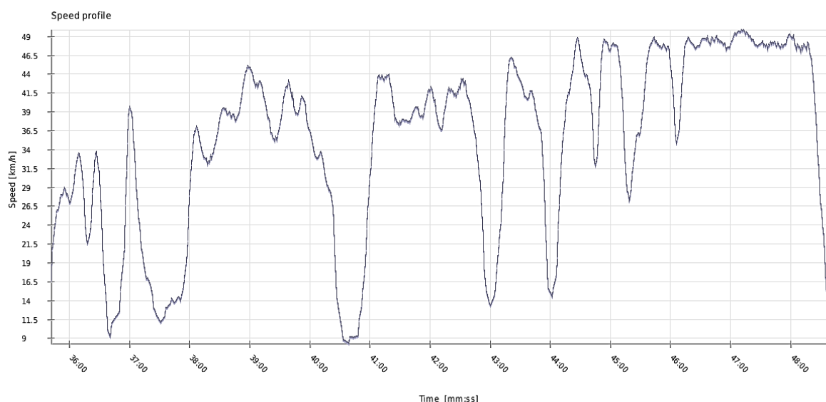
FIGURA 84. VARIAȚIA VITEZEI DE-A LUNGUL TRASEULUI 1 (ALBASTRU) SENS CALEA MOLDOVEI – VIȘOARA
