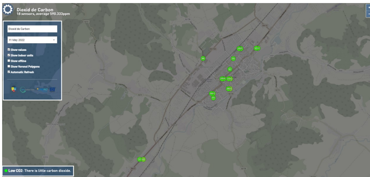
FIGURA 17 LOCAȚIA SENZORILOR DE MONITORIZARE A CALITĂȚII AERULUI ÎN BISTRIȚA (URADMONITOR)
